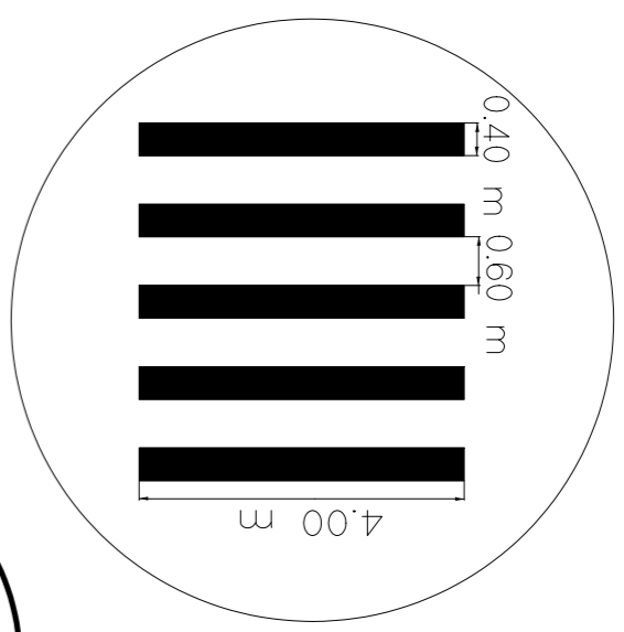
DETALHE 01
